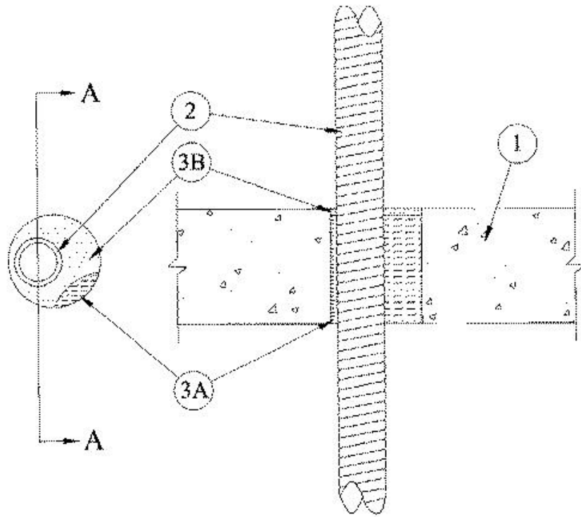
SECTION A-A
